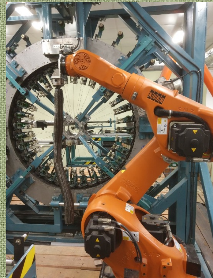
РП-64-6-1-130 KUKA KR-61 6 координат
