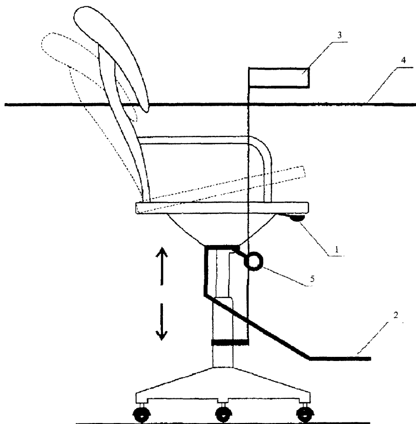
1 - ручное управление изменением высоты и углом наклона
