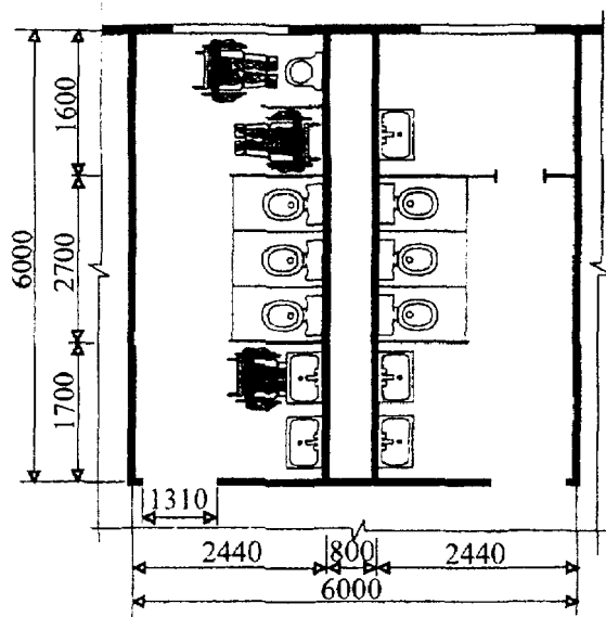
Цеховая уборная с кабиной для инвалидов
