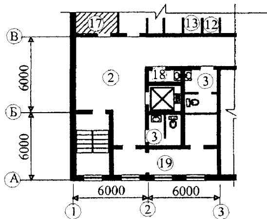
Фрагмент плана на отм. 4.800
