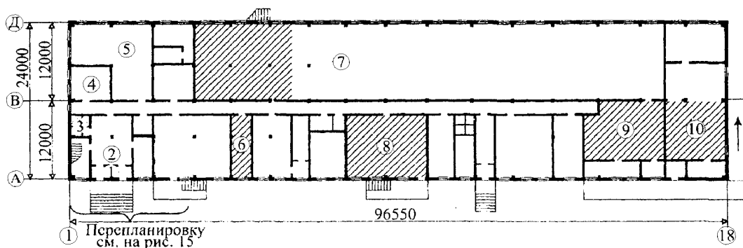
План на отм. 4.800
