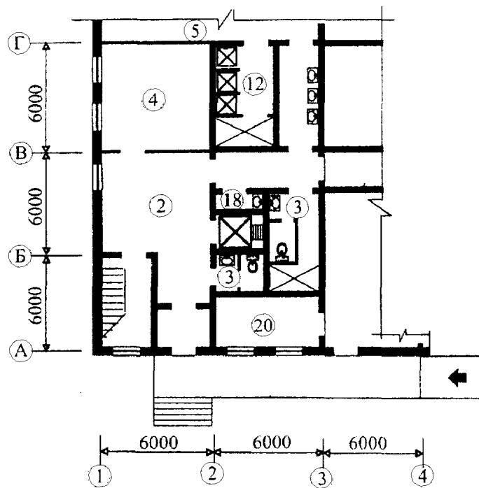
Фрагмент плана на отм. 4.800
